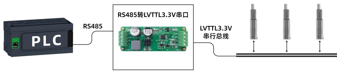
(图 9) PLC 与电缸硬件连接
